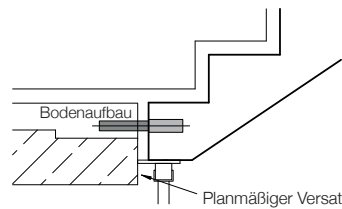
Auflager mit Gewindestangen (ohne Schallschutz)
