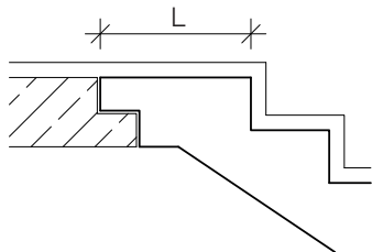
Aufpreis für angeformtes Podest ab einer Länge L \geq 45 \text{ cm}
