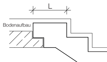
Verlängerter Austritt L > \text{Auftrittsbreite} < 45 \text{ cm}
