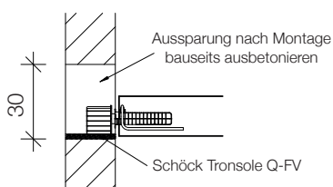
Zwischenaufleger Schöck Q-FV (mit Schallschutz)
