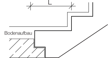
Verlängerter Antritt L > \text{Auftrittsbreite} < 45 \text{ cm}
