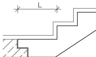
Aufpreis für angeformtes Podest ab einer Länge L \geq 45 \text{ cm}
